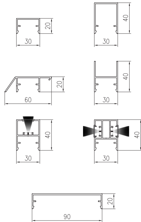
PRZEKRÓJ PRZEZ KLIPSY MASKUJĄCE SYSTEMU VERTILINE
