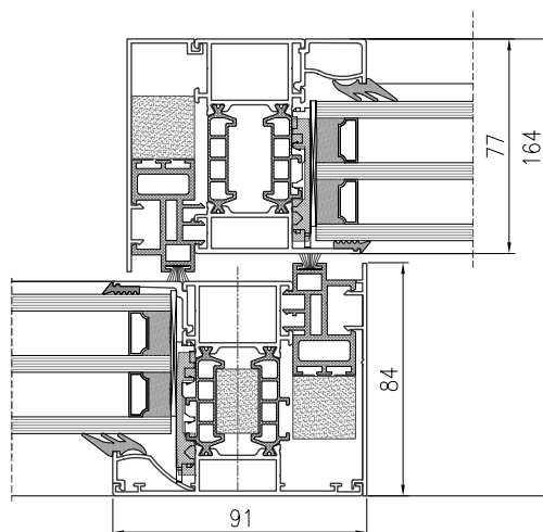
PRZEKRÓJ PRZEZ PRZYMIK NA STYKU ZE ŚCIANĄ PROFILU TM 77HI
